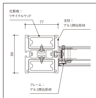
構造図 (HR type/片面表示の図)
